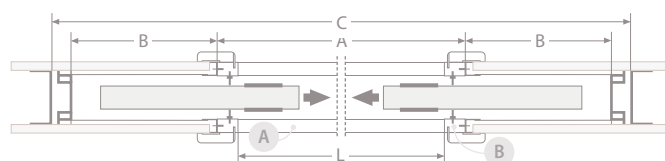
WYMIARY KASETY PODWÓJNEJ (mm)
