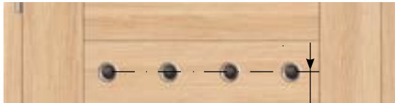
Tuleje wentylacyjne: – szerokość skrzydła „60”, „70” – 4 szt.
