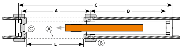
WYMIARY KASETY POJEDYNCZEJ (mm)
